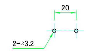
取付穴寸法(リアフィート) Mounting hole dimension (Rear feet)
